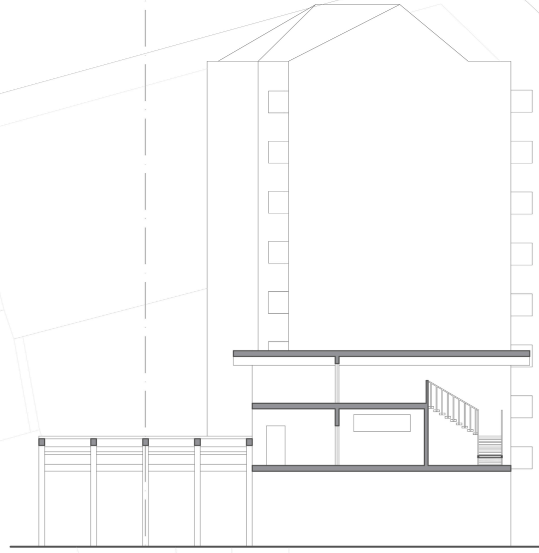
PIANTA A-A'
