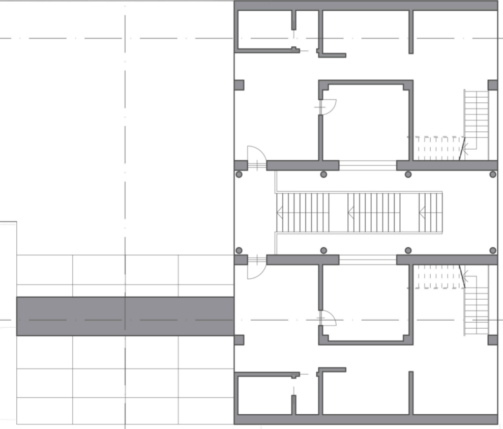
PIANTA C-C'
