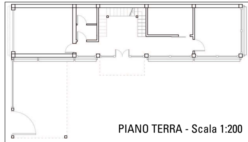
PLANIMETRIA - Scala 1:200
